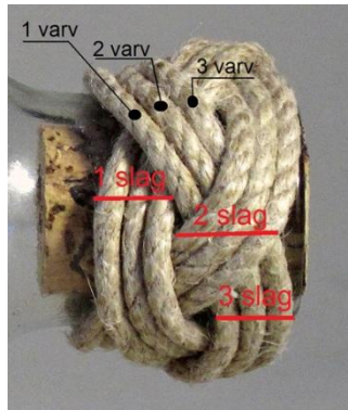
Treslagen valknop
